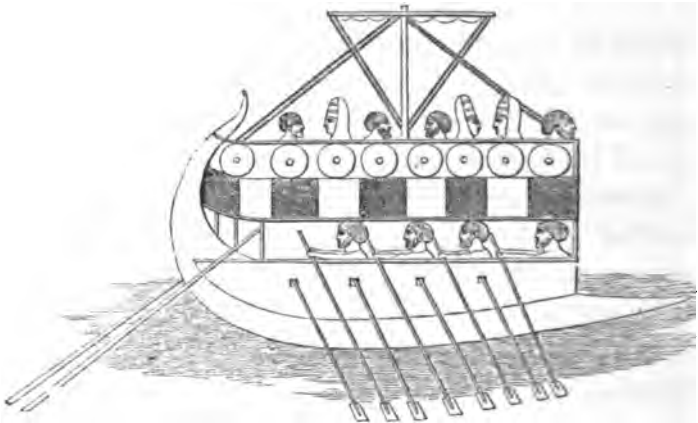
Ship. (Kouyunjik.)
